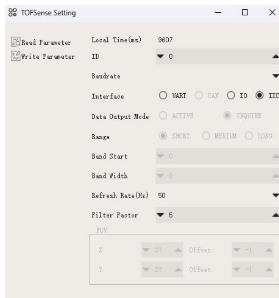
图 3: IIC 输出模式配置图
