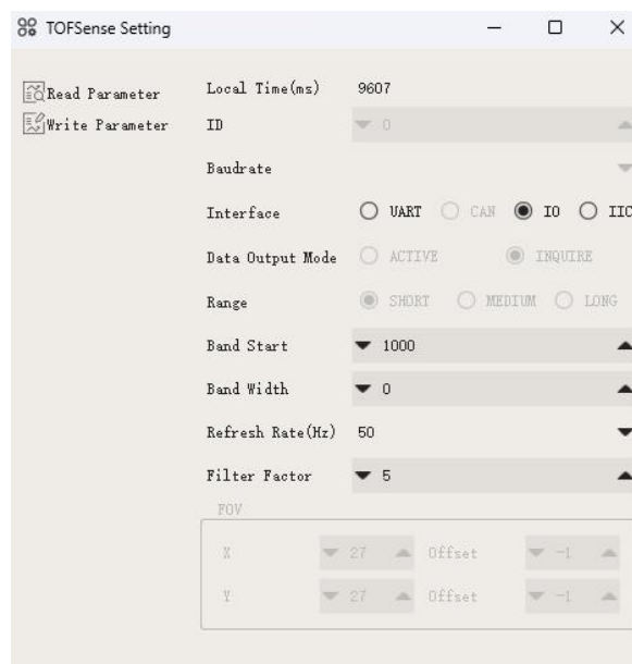
图 4: I/O 模式单阈值设置
