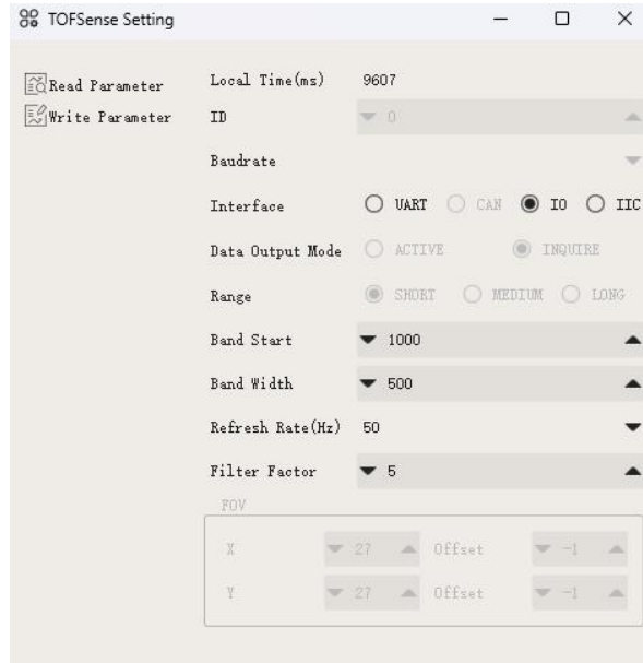
图 5: I/O 模式双阈值设置
