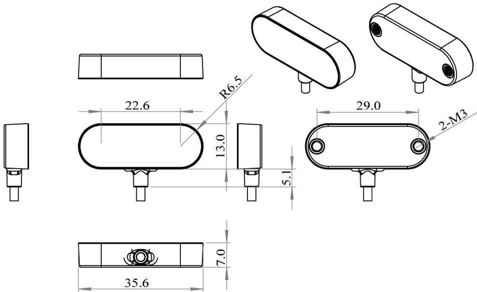
图 8: TOFSense-M S 尺寸图, 单位: mm
