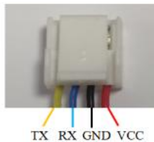
图 3: GH1.25 4P 实际接口线序
