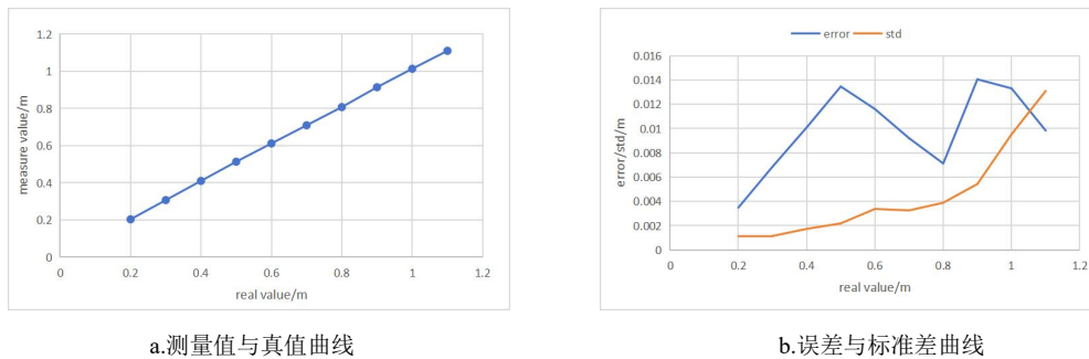
图 6: TOFSense-M 室外 100K LUX 测试结果
