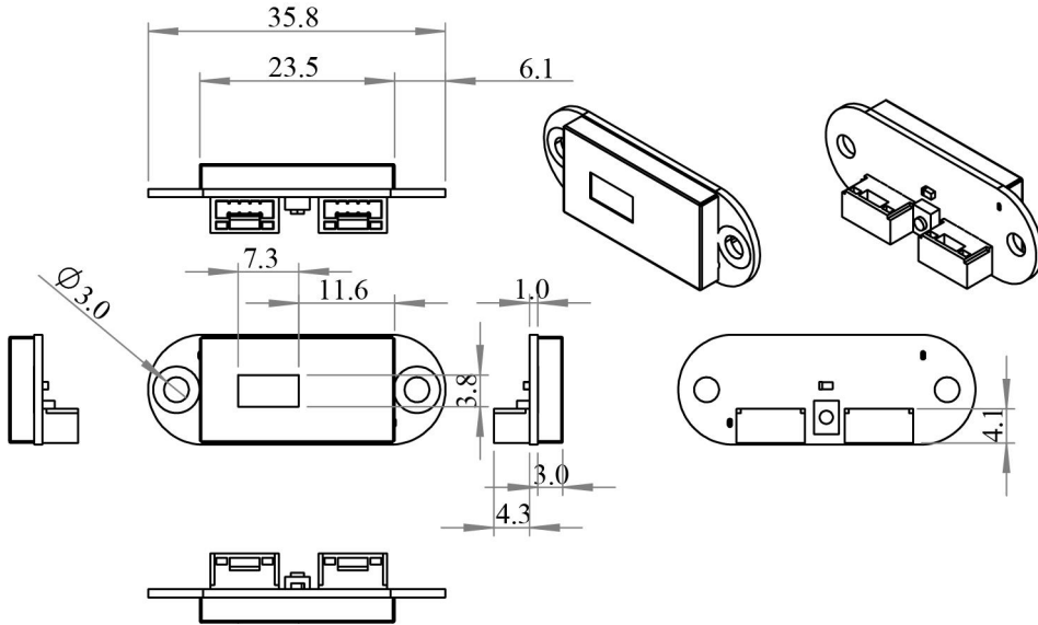
图 7: TOFSense-M 尺寸图, 单位: mm
