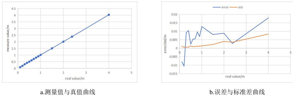
图 5: TOFSense-M 测试结果
