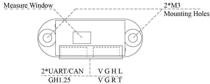
图 1: TOFSense-M 接口
