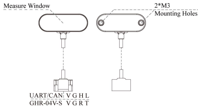
图 2: TOFSense-M S 接口
