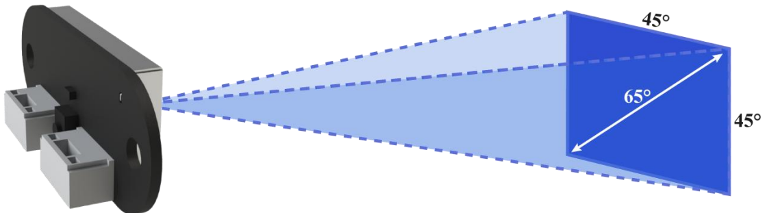
图 5: TOFSense-M 系列 FOV 覆盖区域示意图
