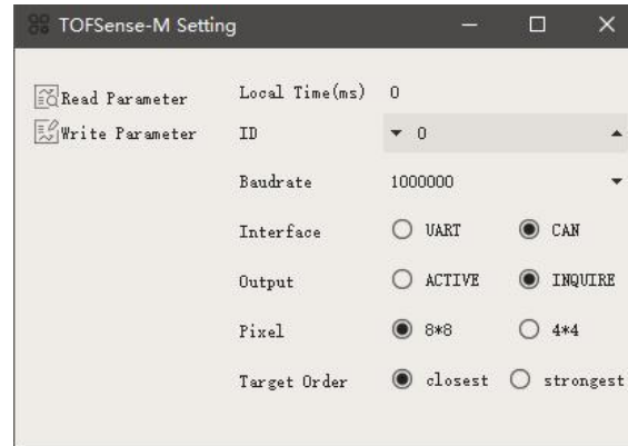
图 4: CAN 查询输出模式配置图
