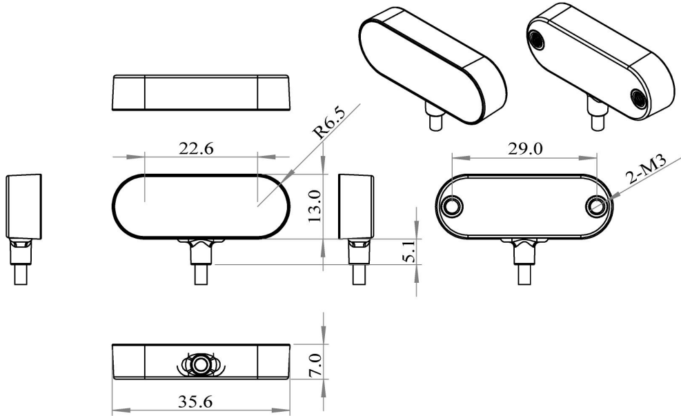
图 9: TOFSense S 尺寸图, 单位: mm
