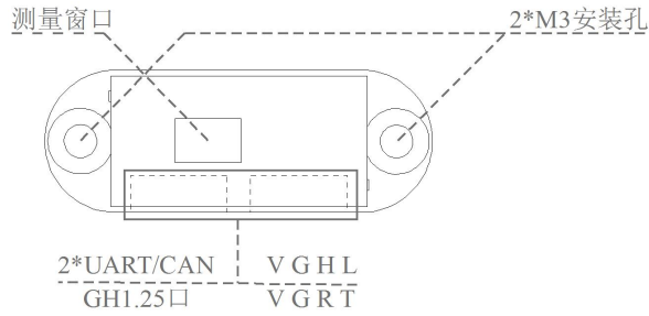
图 1: TOFSense/TOFSense-UART 接口
