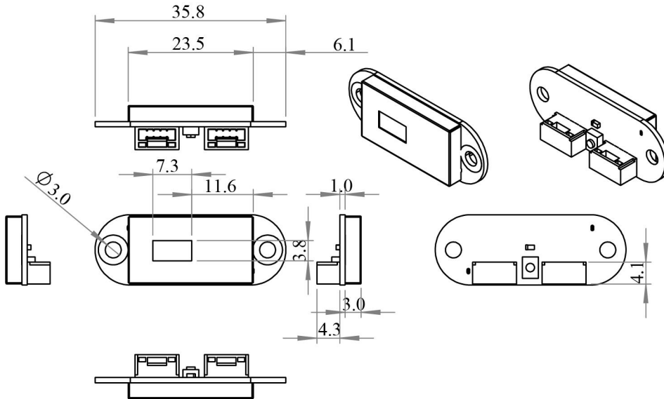
图 8: TOFSense/TOFSense-UART 尺寸图, 单位: mm
