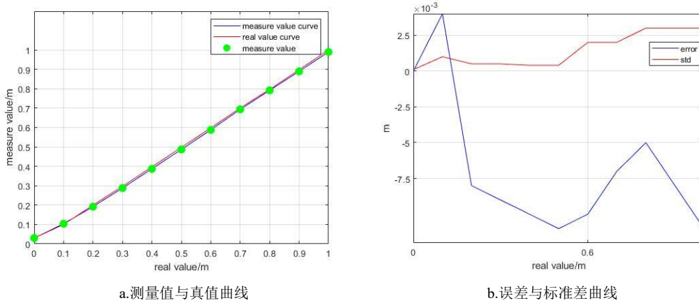
图 7: Short Distance Mode 测试结果
