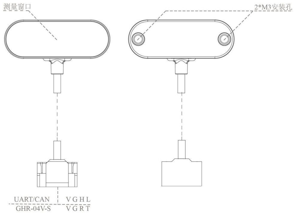
图 2: TOFSense S 接口
