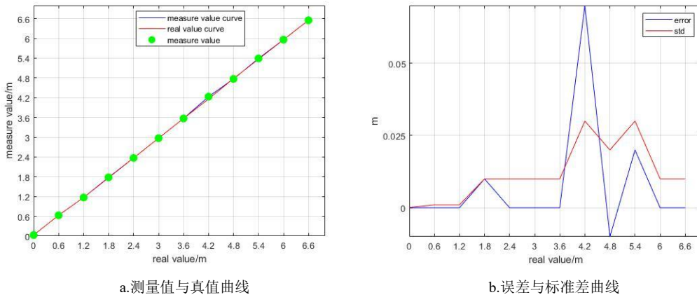
图 6: Medium Distance Mode 测试结果
