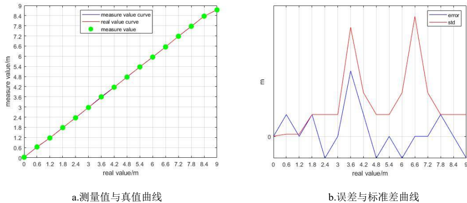
图 5: Long Distance Mode 测试结果
