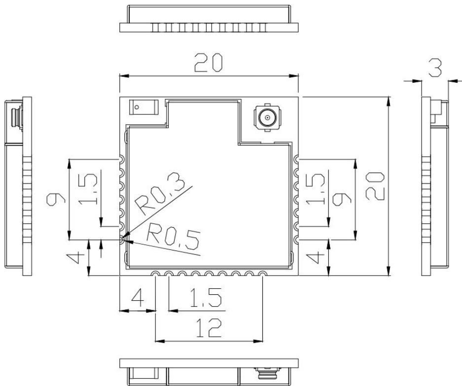
图 2: T06 尺寸图 单位: mm
