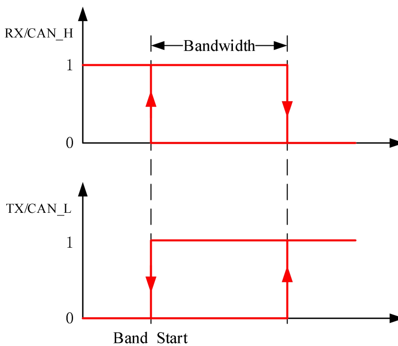
图 6: 滞环比较示意图
