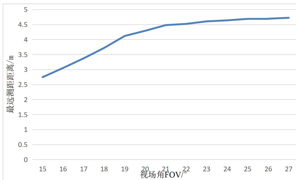
图 10: TOFSense 最远测距距离与视场角 FOV 关系
