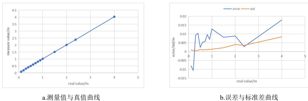
图 4: TOFSense-M S 测试结果
