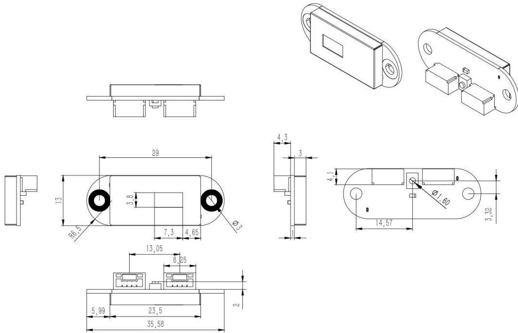
图 6: TOFSense-M 尺寸图, 单位: mm
