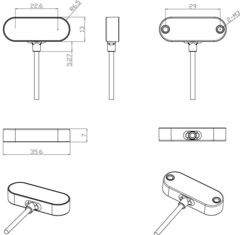
图 7: TOFSense-M S 尺寸图, 单位: mm
