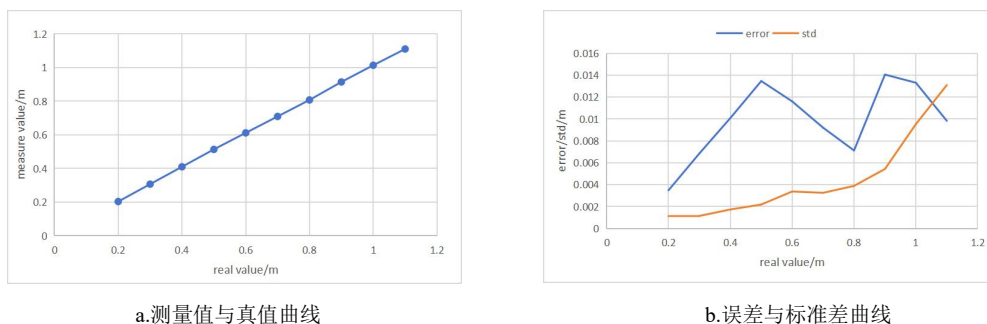
图 5: TOFSense-M S 室外 100K LUX 测试结果
