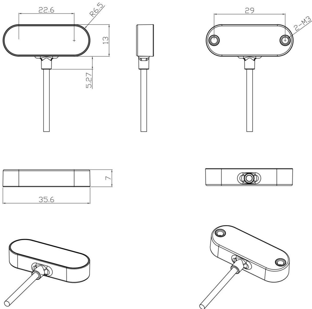
图 6: TOFSense-M S 尺寸图, 单位: mm
