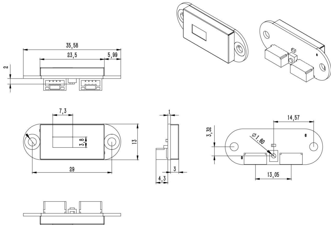
图 5: TOFSense-M 尺寸图, 单位: mm
