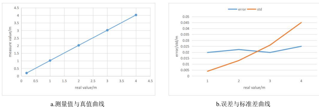
图 4: TOFSense-F 测试结果
