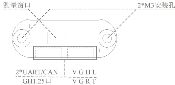
图 1: TOFSense-M 接口
