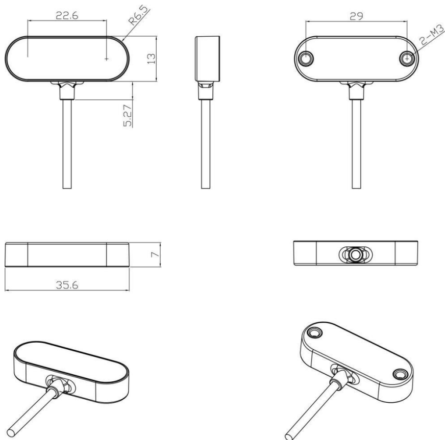
图 6: TOFSense-M S 尺寸图, 单位: mm
