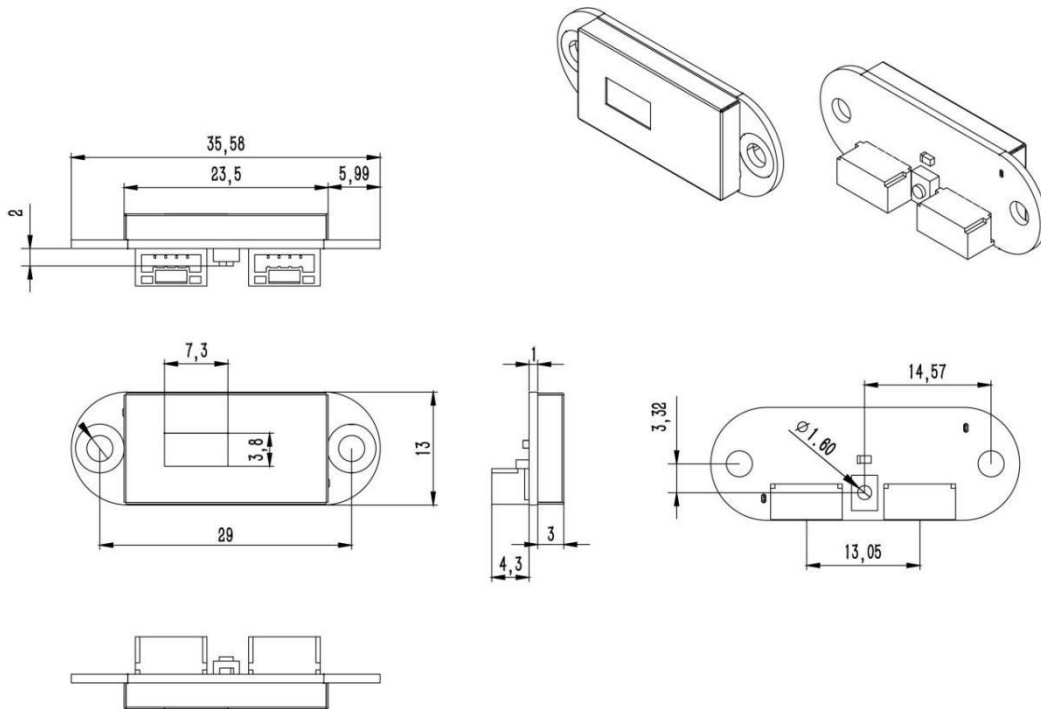
图 5: TOFSense-M 尺寸图, 单位: mm
