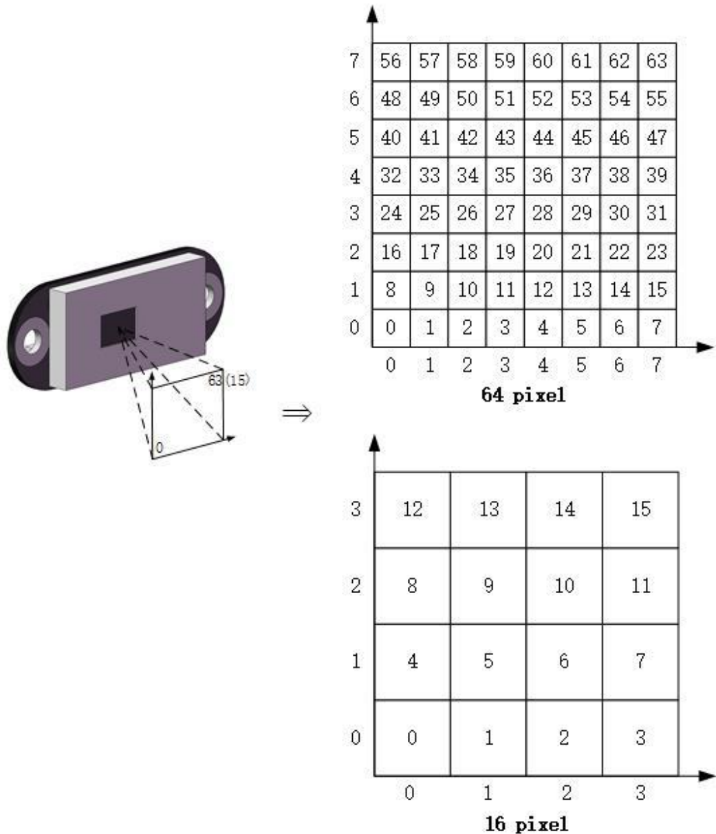
图 5: FOV 与像素点对应示意图
